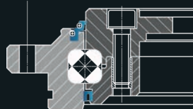
링 스프링 씰링
